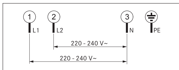
Fig. 5.25 Tilslutningsdiagram 2-faset
