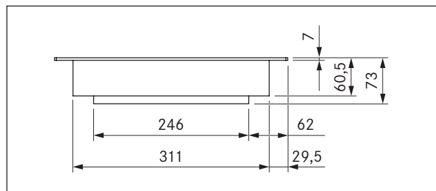
Fig. 3.2 PKT3 apparatmål set forfra
