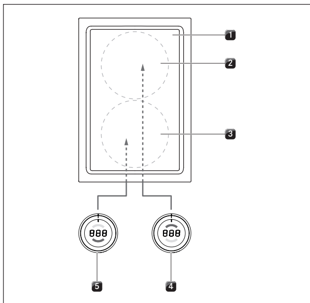
Fig. 5.22 Tilslutning af kogezoner ved indbygning med 180° og ved apparater med tilslutning bagest (PKT3)
