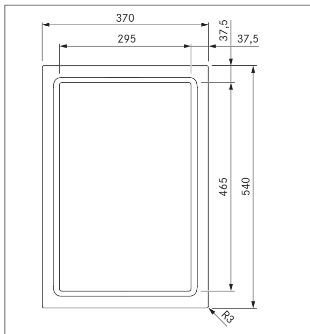
Fig. 3.1 PKT3 apparatmål set fra oven
