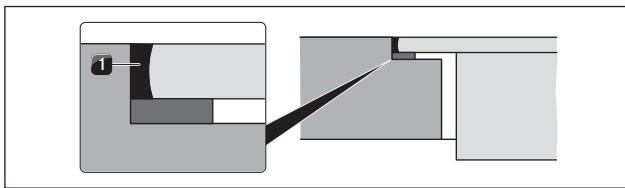
Fig. 5.26 Silikoneforseglingsmasse ved planlimet montering
