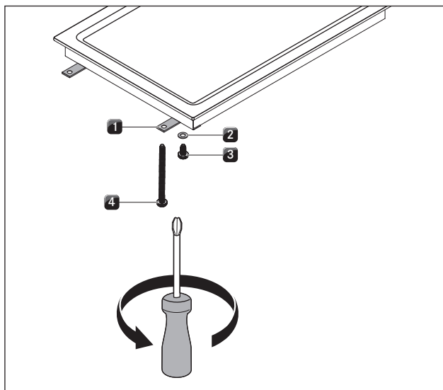
Fig. 5.18 Fastgørelsesclips
