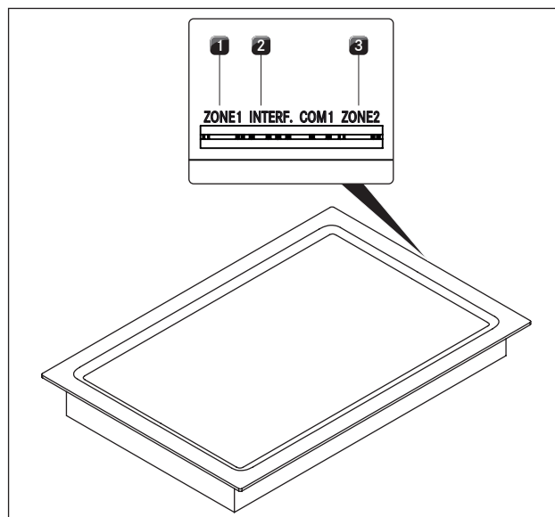
Fig. 5.20 Tilslutning af betjeningsknap på kogepladens bagside
