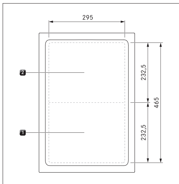
Fig. 4.5 Opbygning af Tepan-grill i rustfrit stål PKT3 og størrelse af kogezone
