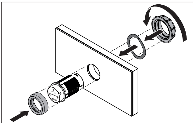
Fig. 5.14 Montering af betjeningsknop
