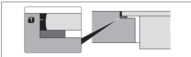
Fig. 5.27 Silikoneforseglingsmasse ved planimet montering
