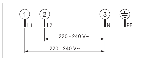
Fig. 5.26 Tilslutningsdiagram 2-faset
